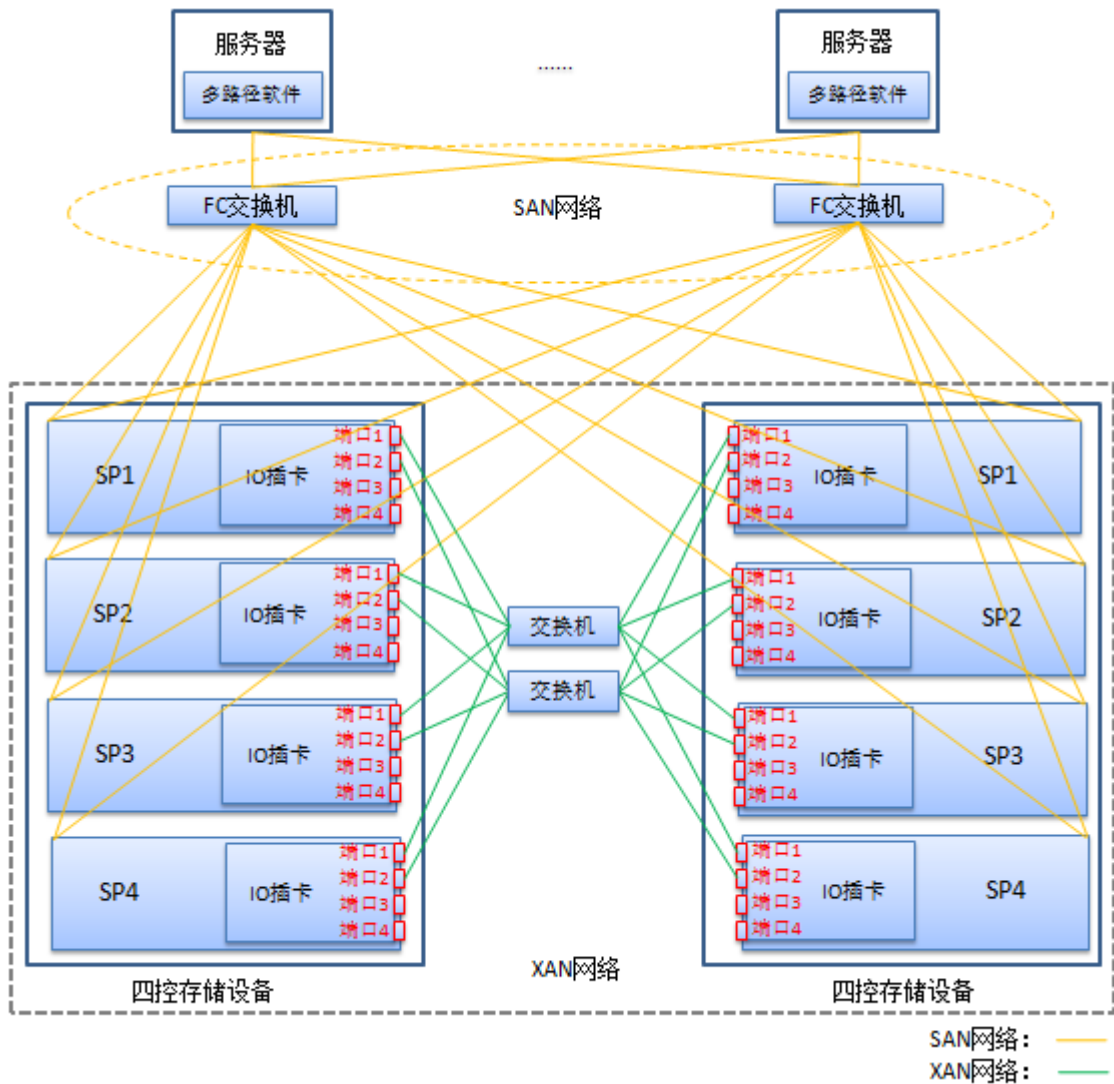
图4-6 四控 XAN 典型组网图（交换机连接）
