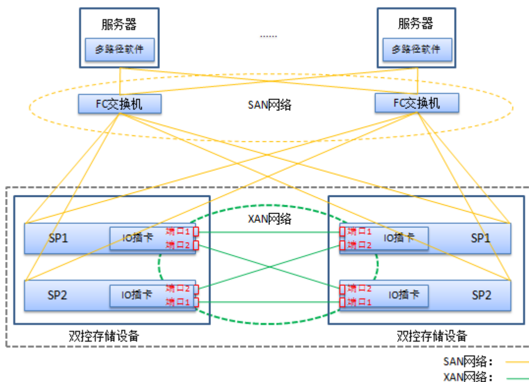
图4-3 双控 XAN 典型组网图 (MESH 直连)
