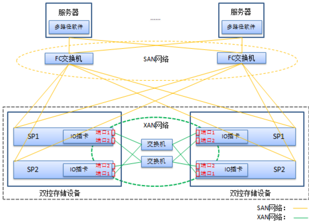
图4-4 双控 XAN 典型组网图（交换机连接）
