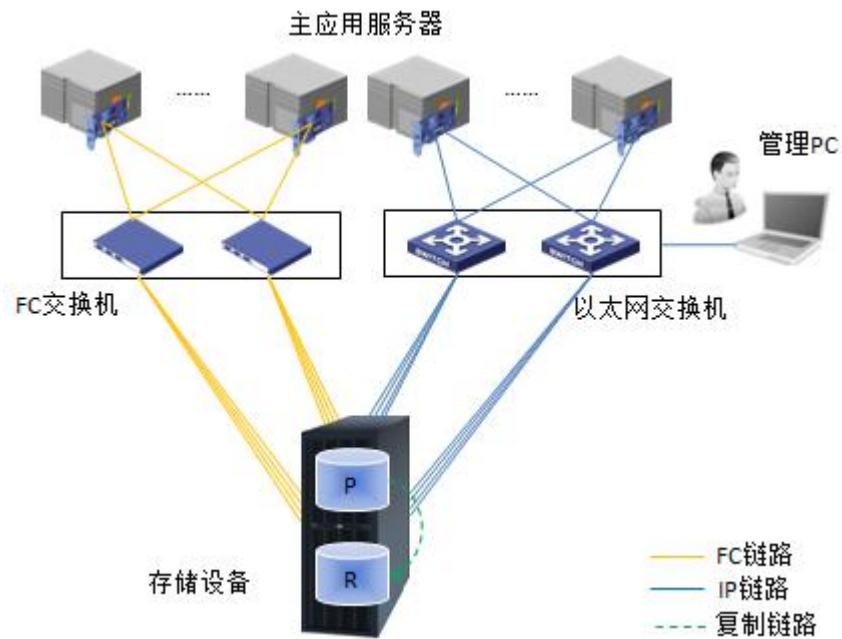
图4-1 本地复制典型组网图
