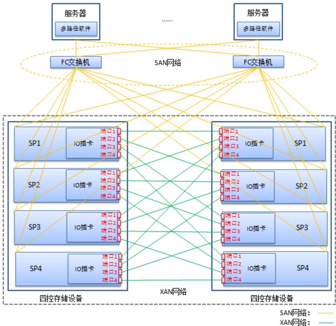
图4-5 四控 XAN 典型组网图（MESH 直连）
