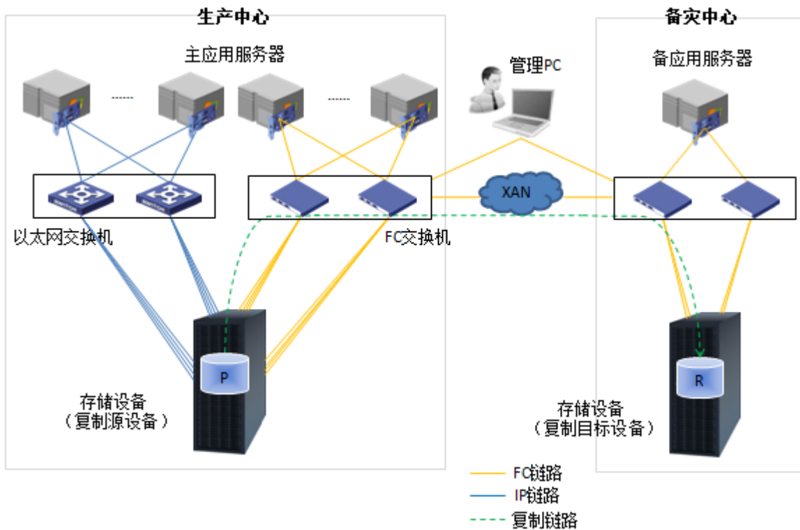
图4-2 远程复制典型组网图
